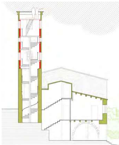
Secció reformada de la torre.
