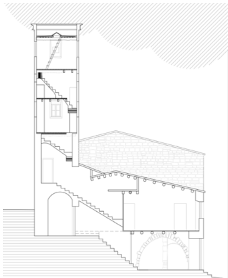
Secció existent de la torre.
